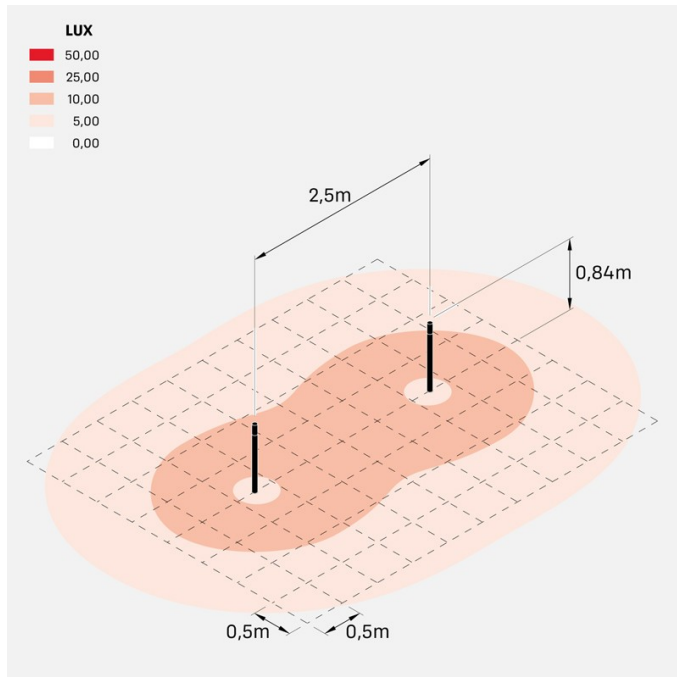
stik_60_opal_bollard_840
