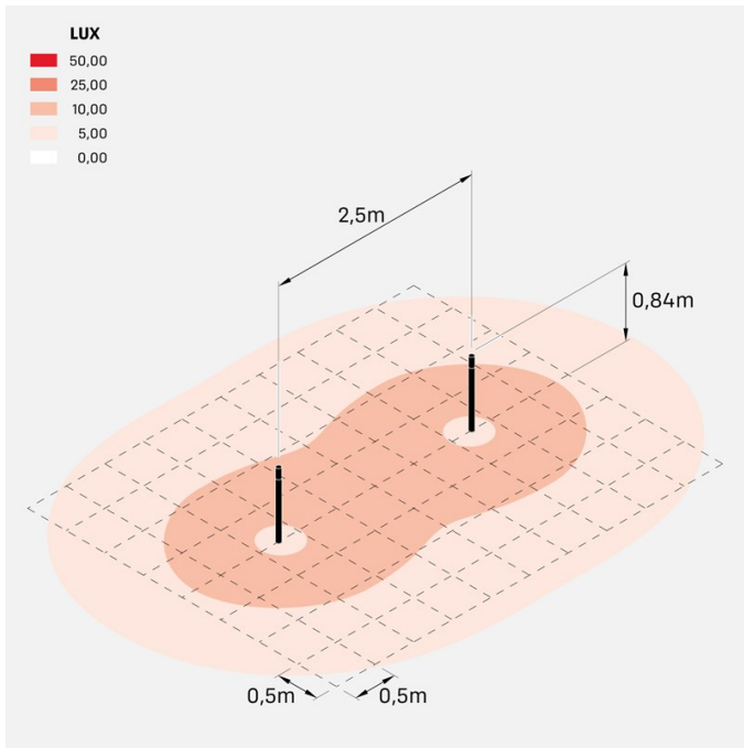
stik_60_opal_bollard_840
