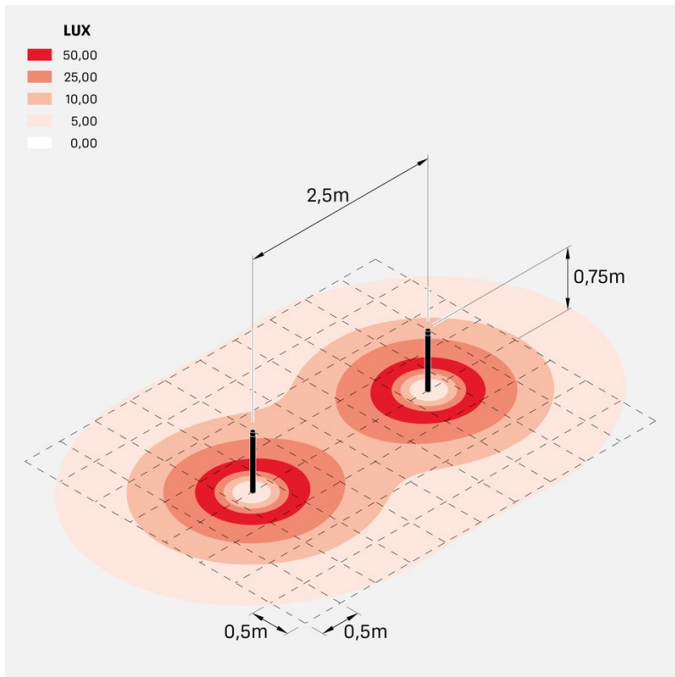
stik_60_flat_trasp_bollard_750
