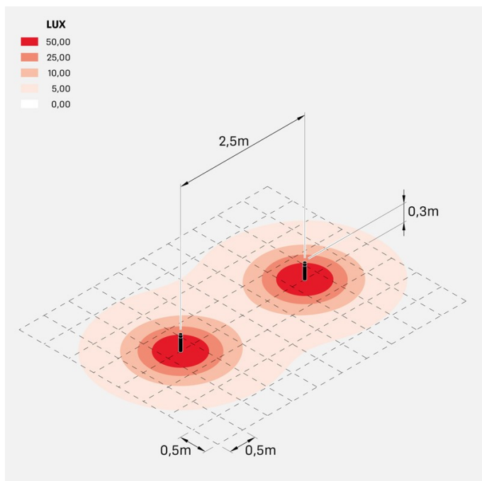
stik_60_flat_opal_bollard_300
