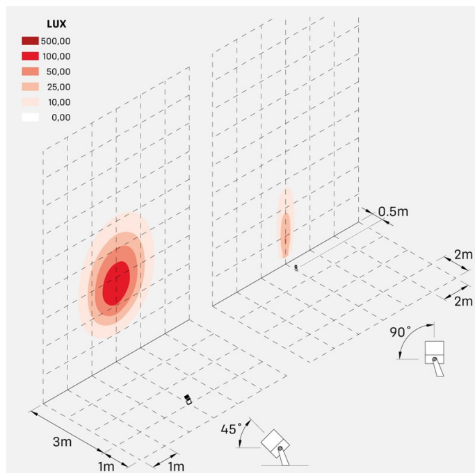
pad_mini_optic_M
