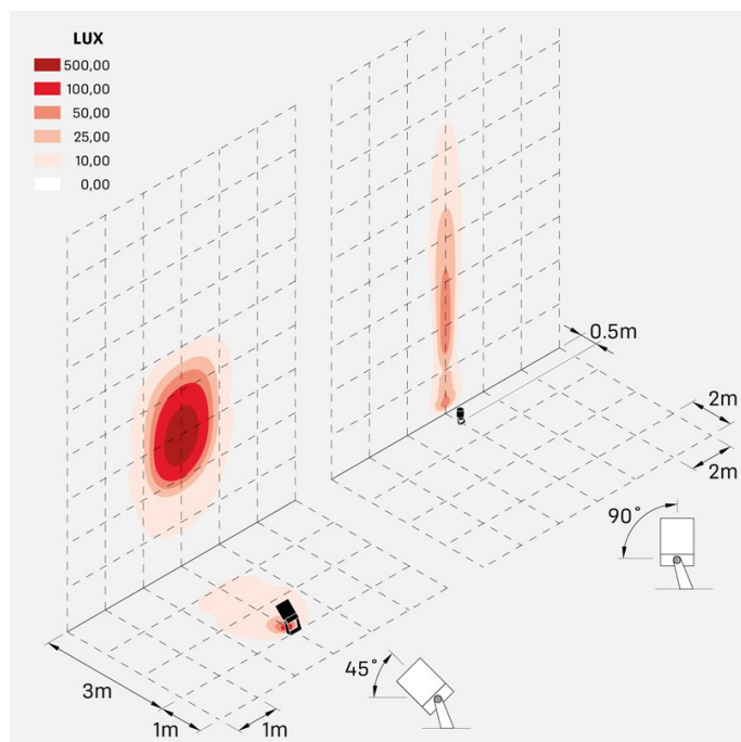
pad_maxi_rgbw_optic_S
